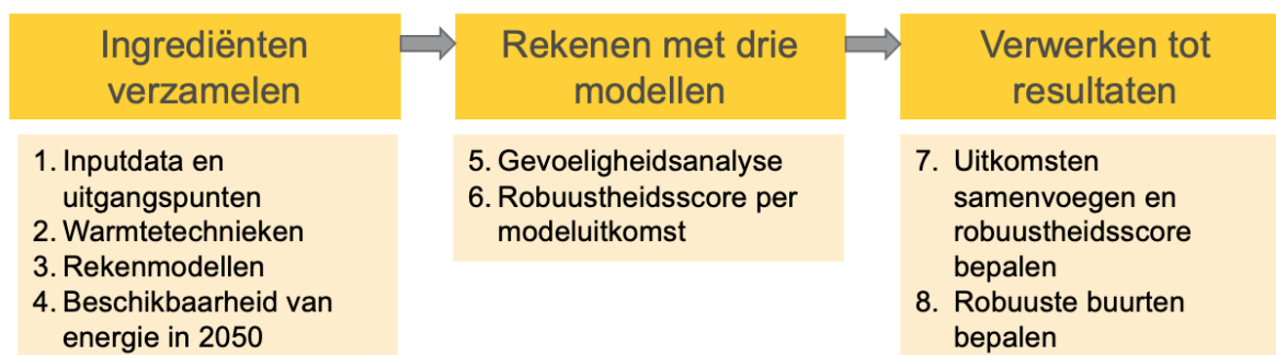
Figuur 1 - Modelleerstappen
