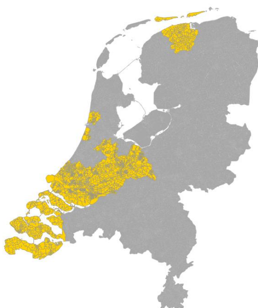
Figuur 2 - Rekengebied
