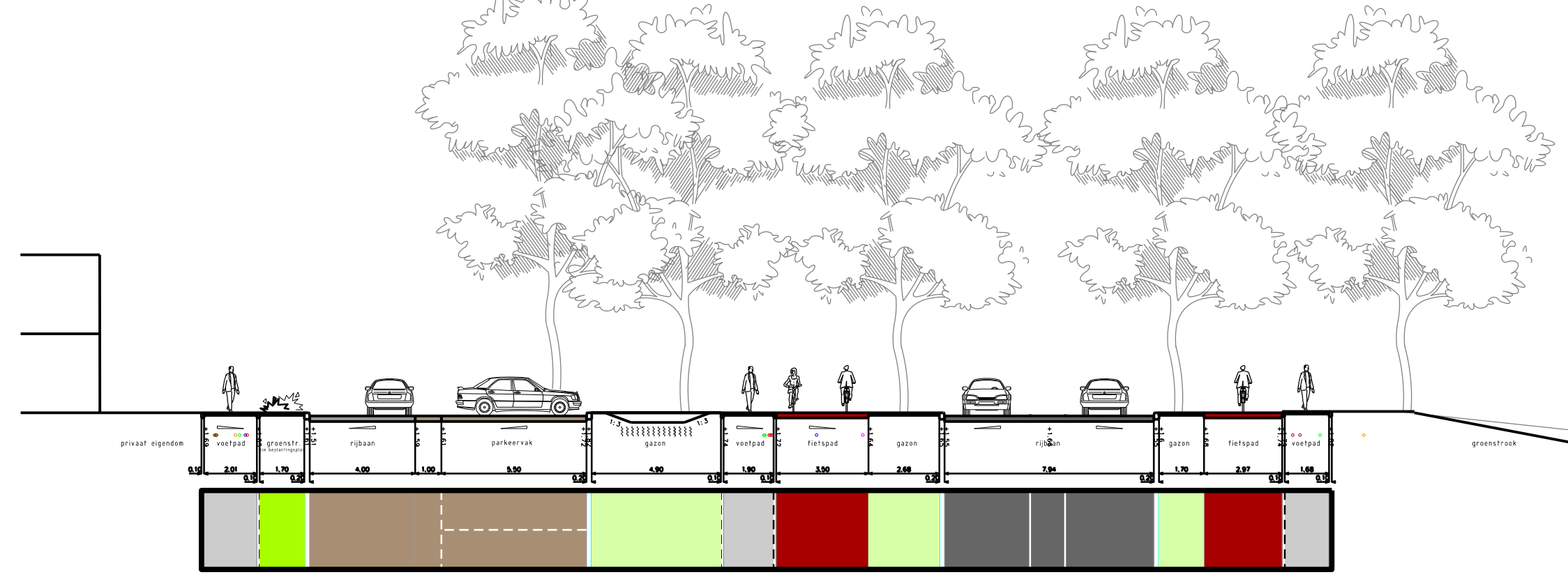
Profiel D-D'
