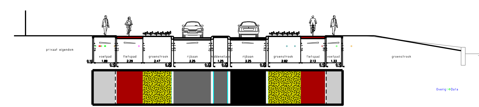
Profiel A-A'
