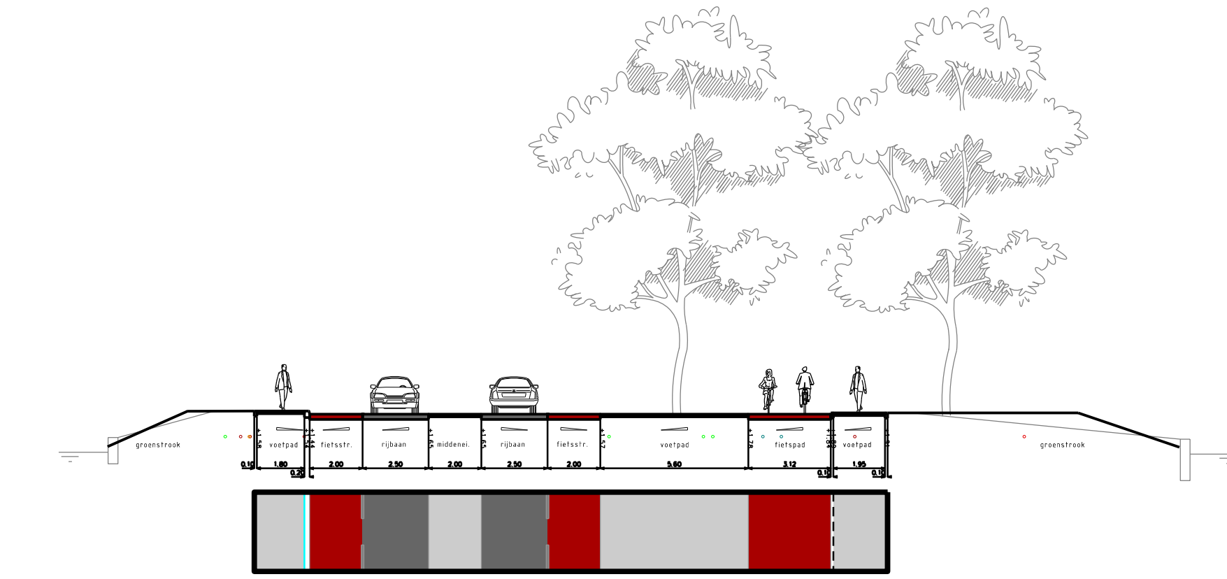
Profiel B-B'
