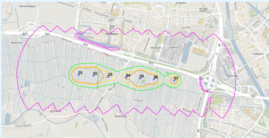
figuur 3: contouren zonder meest oostelijke turbine (groen: L_{den} 45 dB, geel: L_{den} 47 dB, oranje: L_{night} 41 dB, paars: L_{night} 40 dB)
