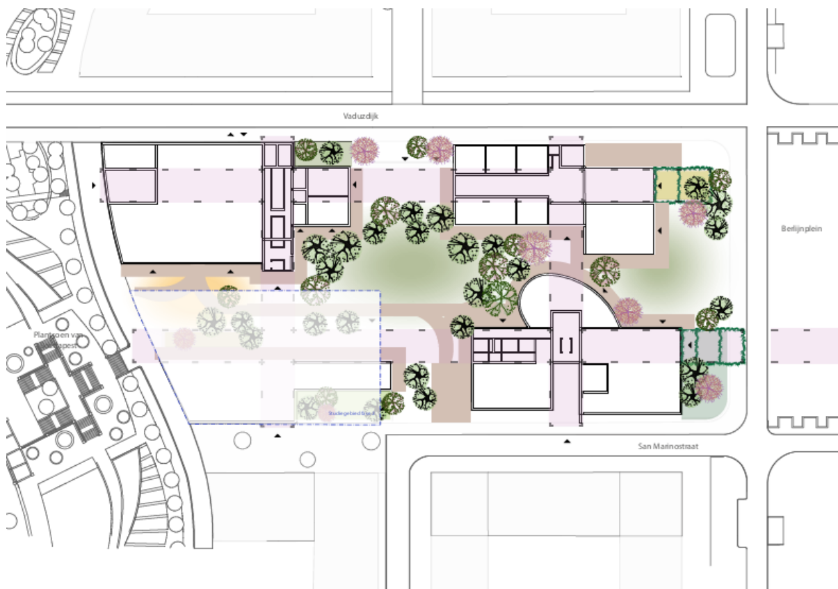
Afbeelding 2: Plattegrond SO
