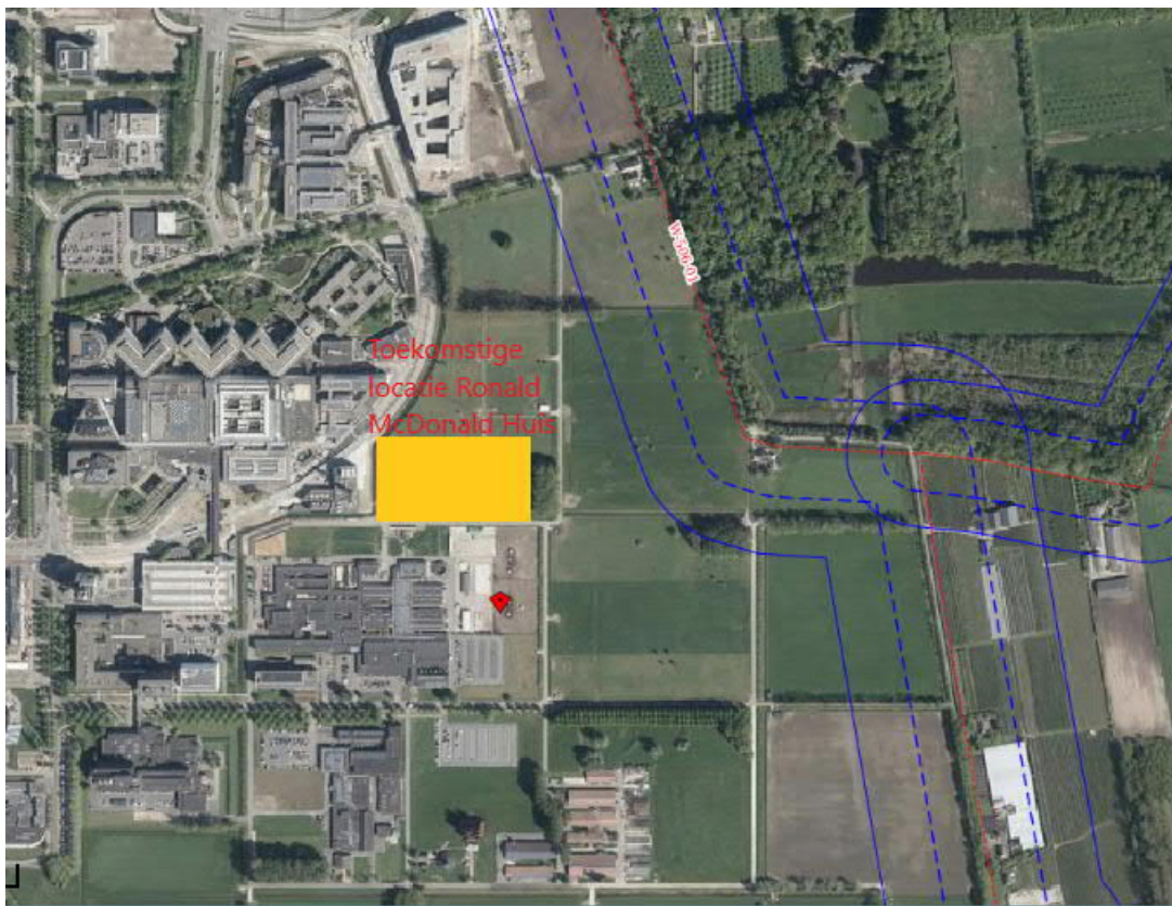
Figuur 4-3 Veiligheidsafstanden hogedrukaardgasleiding
